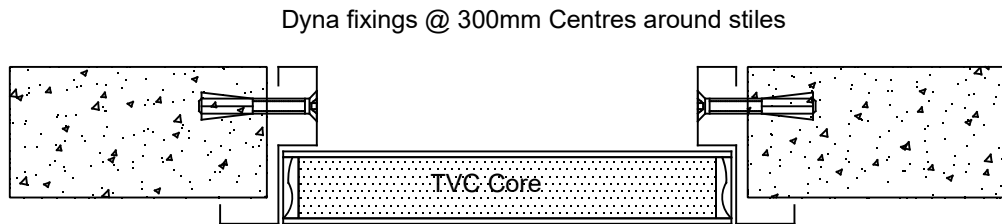
ELEVATION
