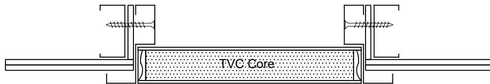
ELEVATION
